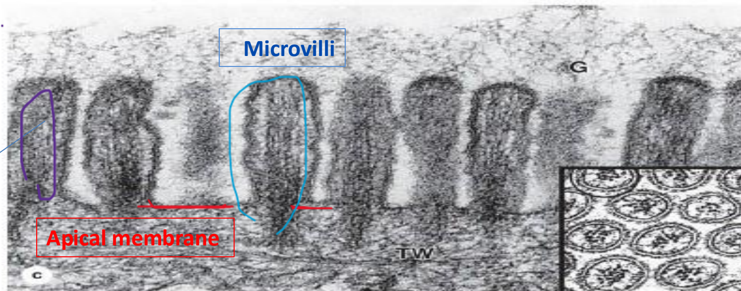
TEM
