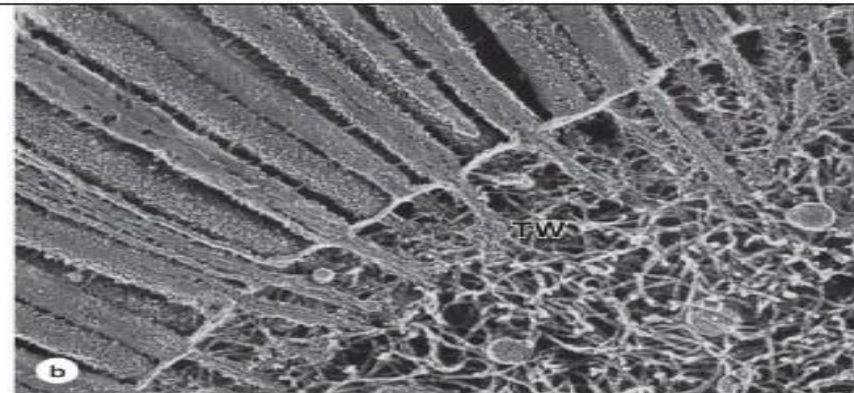
SEM
